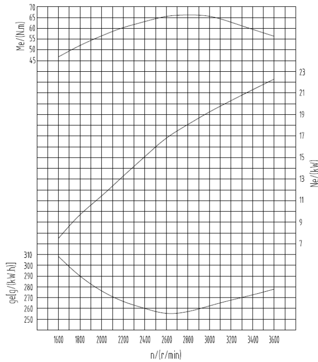
2V95外特性曲线
